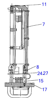
Schnitt A-A Section A-A
